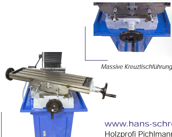
Kreuztisch schwenkbar
