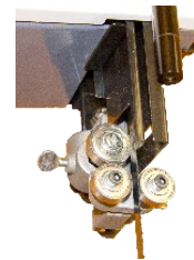
Kugelgelagerte Bandführung
